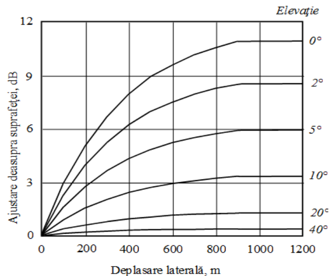
Figura 2.7.o: Variația atenuării laterale \Lambda(\beta, \ell) cu unghiul de elevație și distanța
