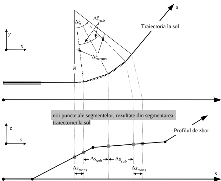
Figura 2.7.f: Construcția segmentelor traiectului de zbor prin divizarea virajului în segmente de lungimea \Delta s (sus – vedere în plan orizontal, jos – vedere în plan vertical)
