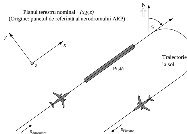
Figura 2.7.b: Sistemul de coordonate locale și (x,y,z) coordonata fixă s a traiectoriei la sol
