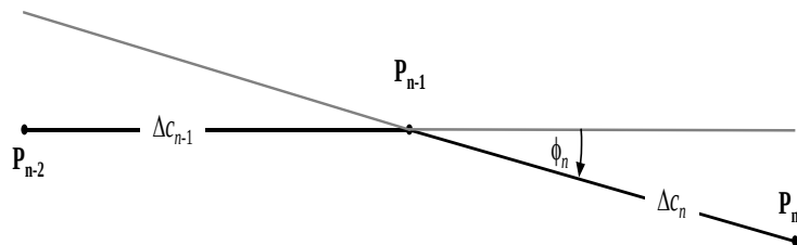
Figura 2.7.v: Parametrii geometrici care definesc șirul șirul algoritmului de trasare
