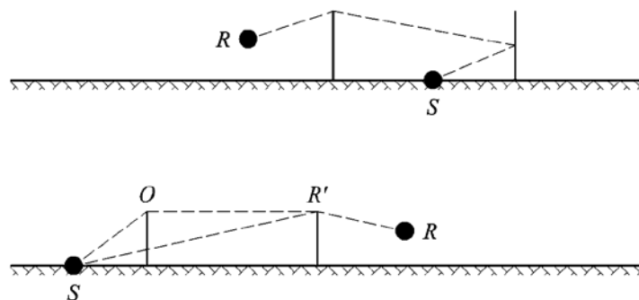
Figura 2.5.j: Diferența traiectoriei în prezența unei difracții: secțiunea transversală actuală (partea superioară), secțiunea transversală nedesfășurată (partea inferioară) În cazul reflexiilor multiple se adaugă reflexiile datorate fiecărei reflexii.
