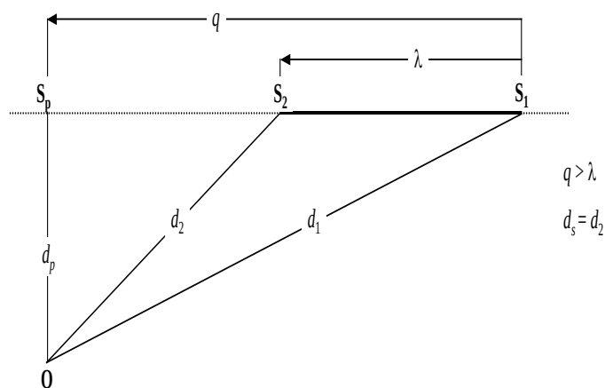
Figura 2.7.1: Geometria segmentului traiectului de zbor pentru poziția observatorului înaintea segmentului
