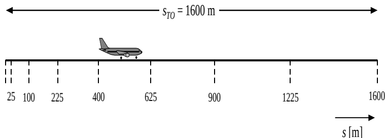
Figura 2.7.g: Segmentarea rulării pentru decolare (exemplu cu 8 segmente)
