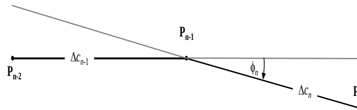
Figura 2.7.v: Parametrii geometrici care definesc șirul șirul algoritmului de trasare
