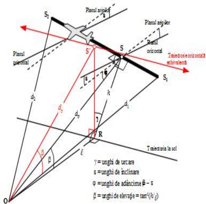
Figura 2.7.p : Observatorul în dreptul segmentului
