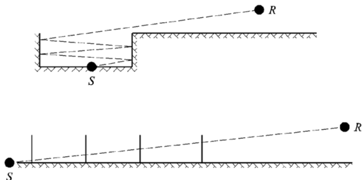
Figura 2.5.h: Unda de sunet reflectată la ordinul de 4 pe o linie aflată într-un șanț: secțiunea transversală actuală (partea superioară), secțiunea transversală nedeșfășurată (partea inferioară)
