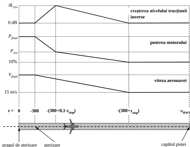
Figura 2.7.h: Modelarea rulării la sol pentru aterizare
