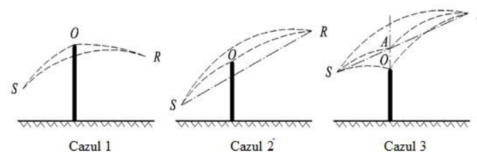
Figura 2.5.e: Calculul diferenței traiectoriei în condiții favorabile (difracție unică) În condiții favorabile, se consideră că cele trei unde sonore curbate SO, OR și SR au o rază de curbare identică \Gamma definită de:
