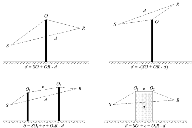
Figura 2.5.d: Calculul diferenței traiectoriei în condiții omogene. O, O1 și O2 sunt punctele de difracție Notă: Pentru fiecare configurare, este dată expresia \delta . Condiții favorabile
