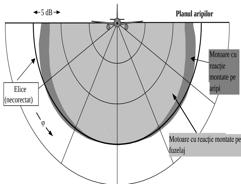
Figura 2.7.n: Directivitatea laterală a efectelor amplasării
